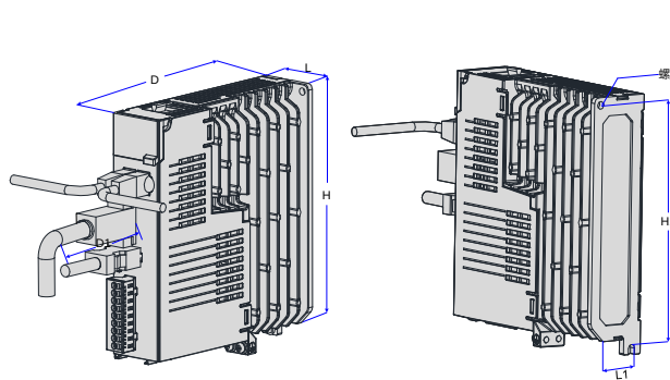
SIZE A 驱动器外形尺寸图
