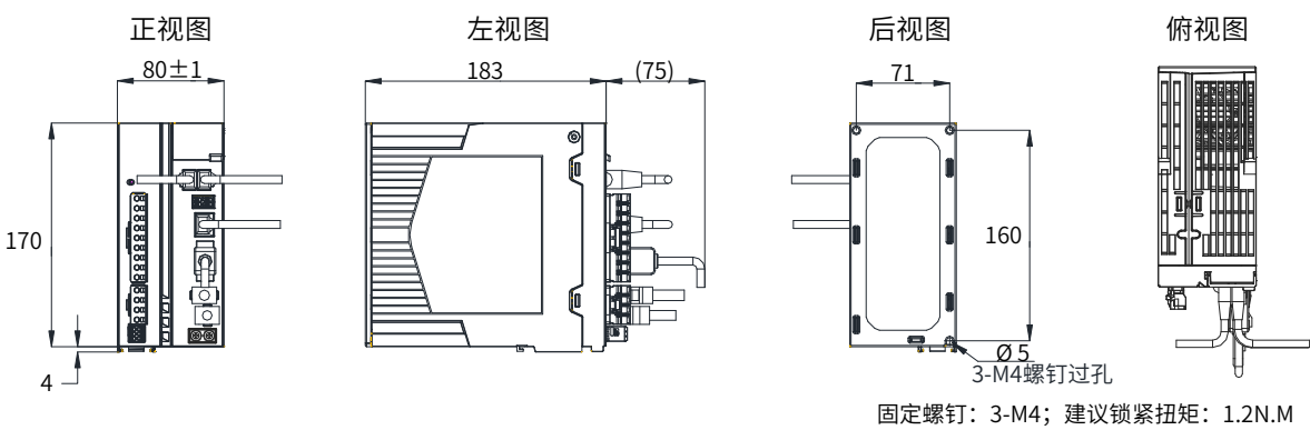
SIZE E 驱动器外形尺寸图
