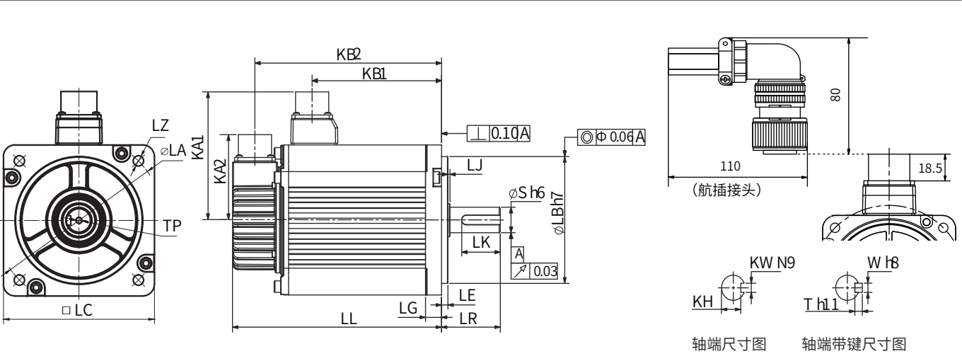
MS1H2（Vn=3000rpm，Vmax=6000/5000rpm）系列外形尺寸图（单位：mm）
