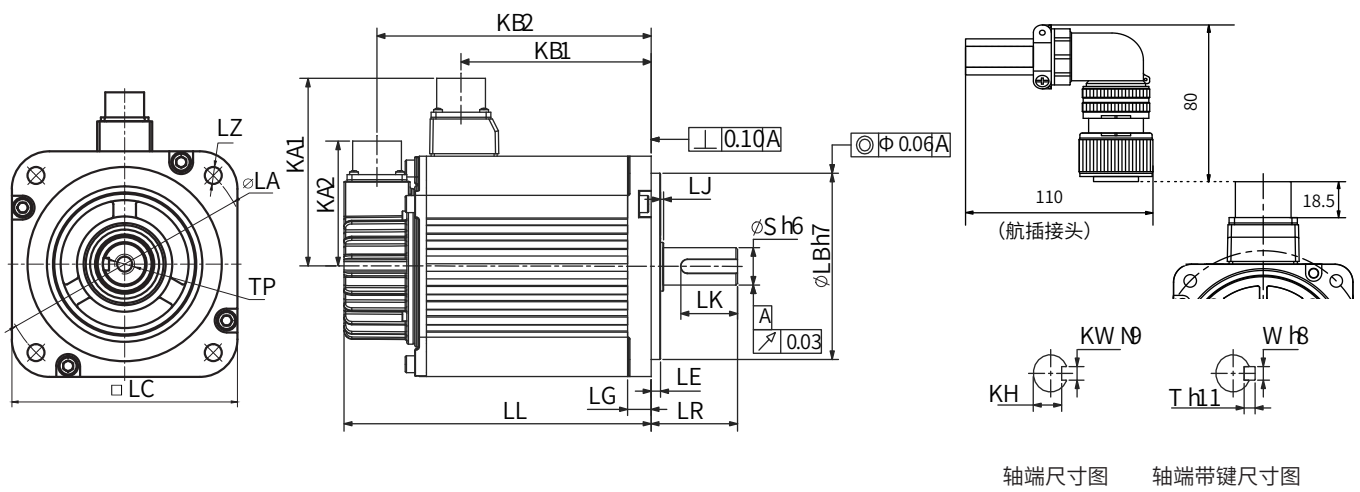
MS1H3（Vn=1500rpm，Vmax=3000rpm）系列外形尺寸图（单位：mm）
