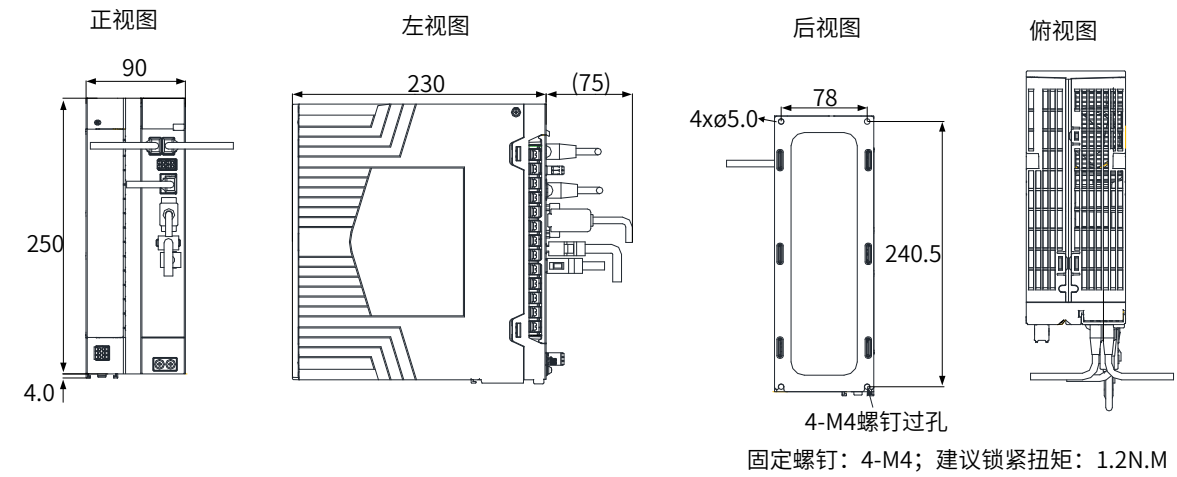
SIZE E 驱动器外形尺寸图
