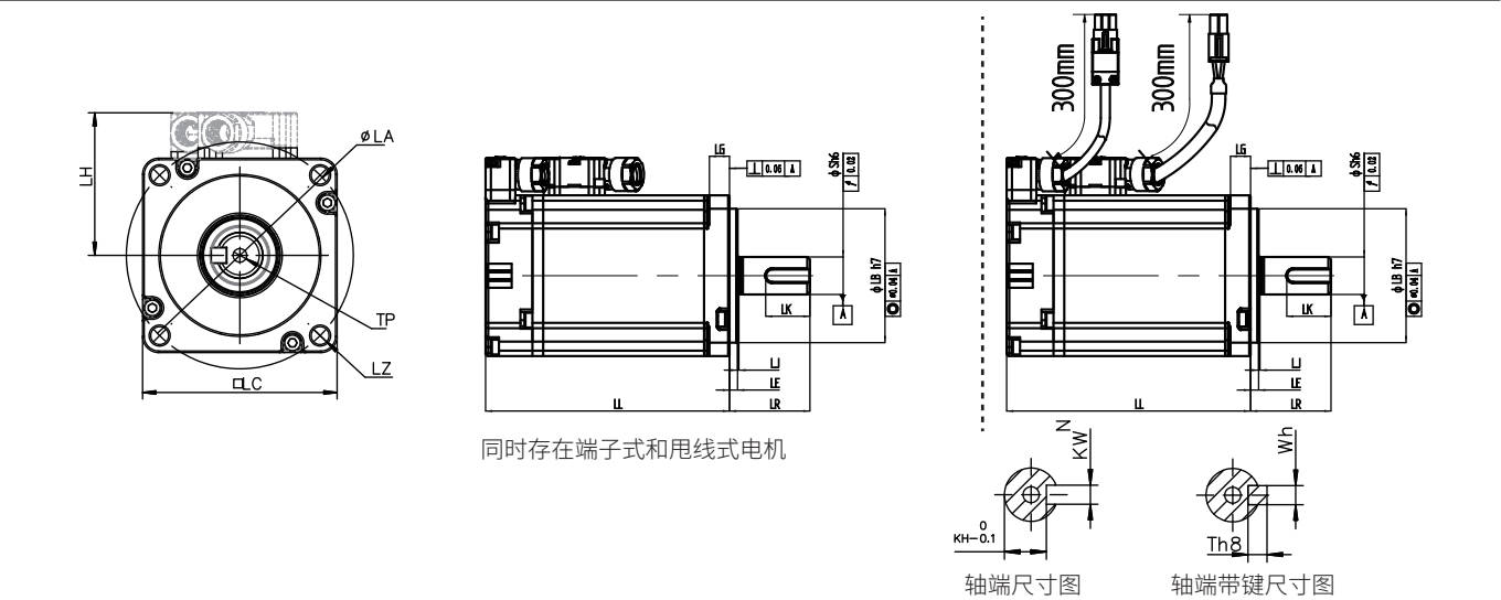
MS1H1（Vn=3000rpm，Vmax=6000rpm）系列外形尺寸图（单位：mm）
